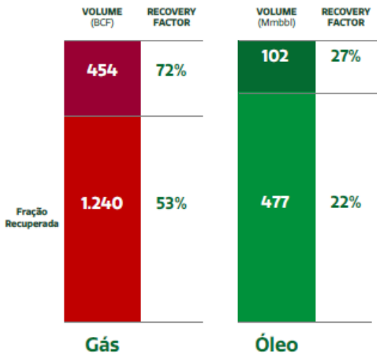
Gráfico 6 – Produção de Óleo e Gás
