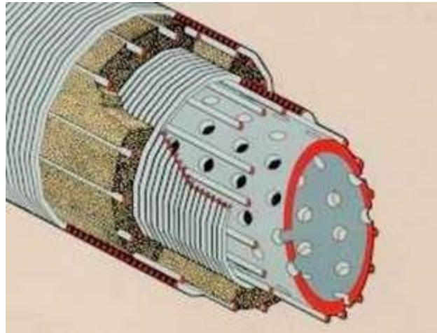
Imagem 12 - Ilustração do processo de canhoneio
