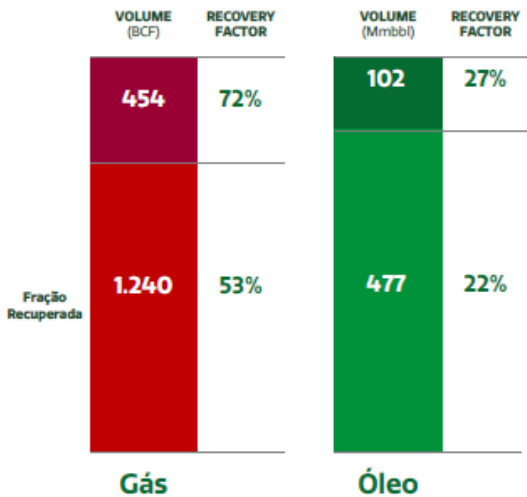
Gráfico 6 – Produção de Óleo e Gás
